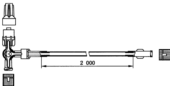
图 D.1 测定丸剂体积的试验装置
